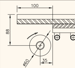
OPTIONAL INFED ROLLER
