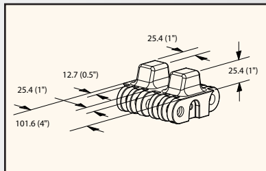
T1 DIMENSIONS
