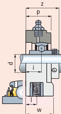
Versión con rodamiento inox YAR 2RF
