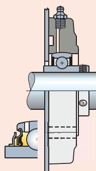
Versión con rodamiento inox YAR 2RF
