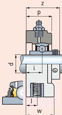
Versión con rodamiento YAR 2F
