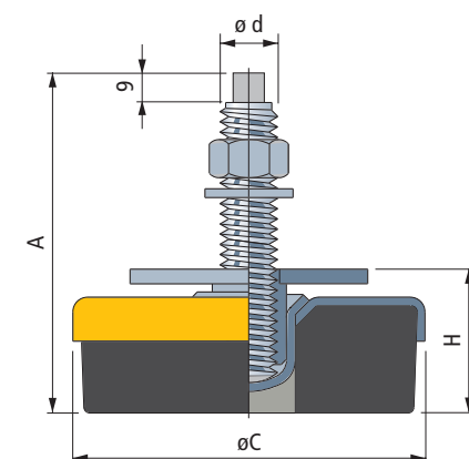
Componentes del pie
