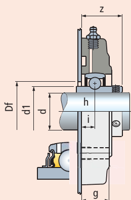
Versión con rodamiento YAR 2F
